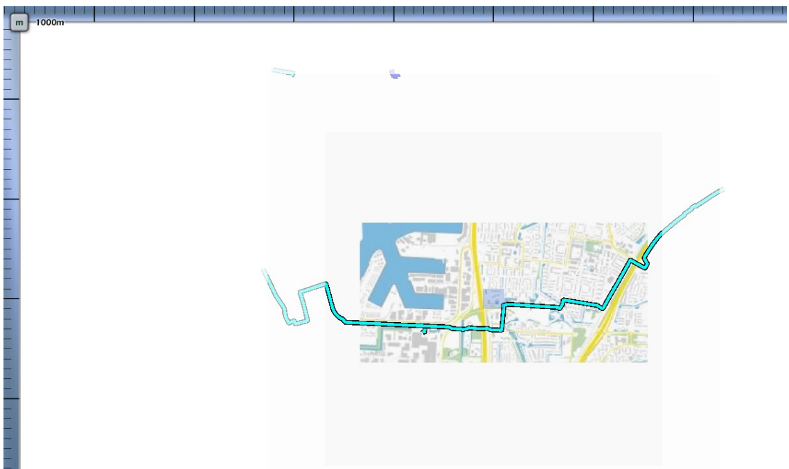
3.2 Figuur 3.2 Plaatsgebonden risico voor 9444_leiding-W-507-03-deel-1 van N.V. Nederlandse Gasunie
