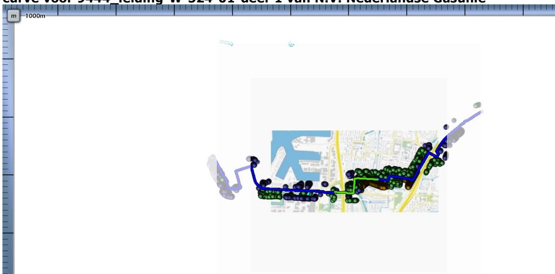
Figuur 4.4 Kilometer leiding behorende bij de maximale overschrijding van de FN-curve voor 9444 leiding-W-524-01-deel-1 van N.V. Nederlandse Gasunie
