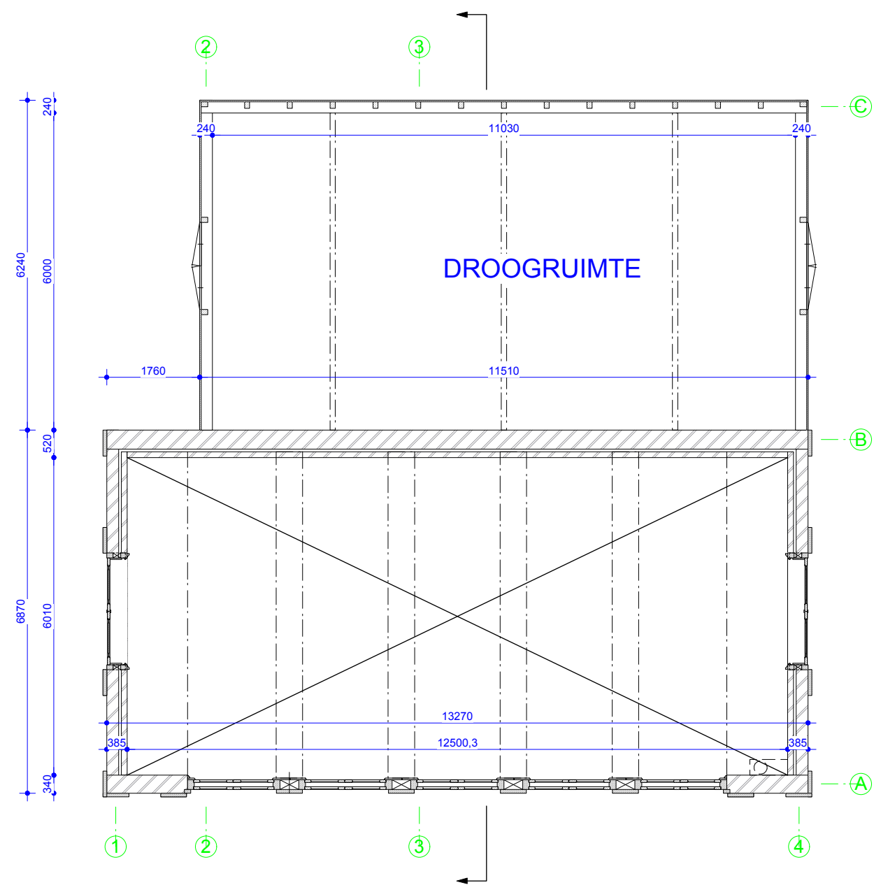
VERDIEPING
