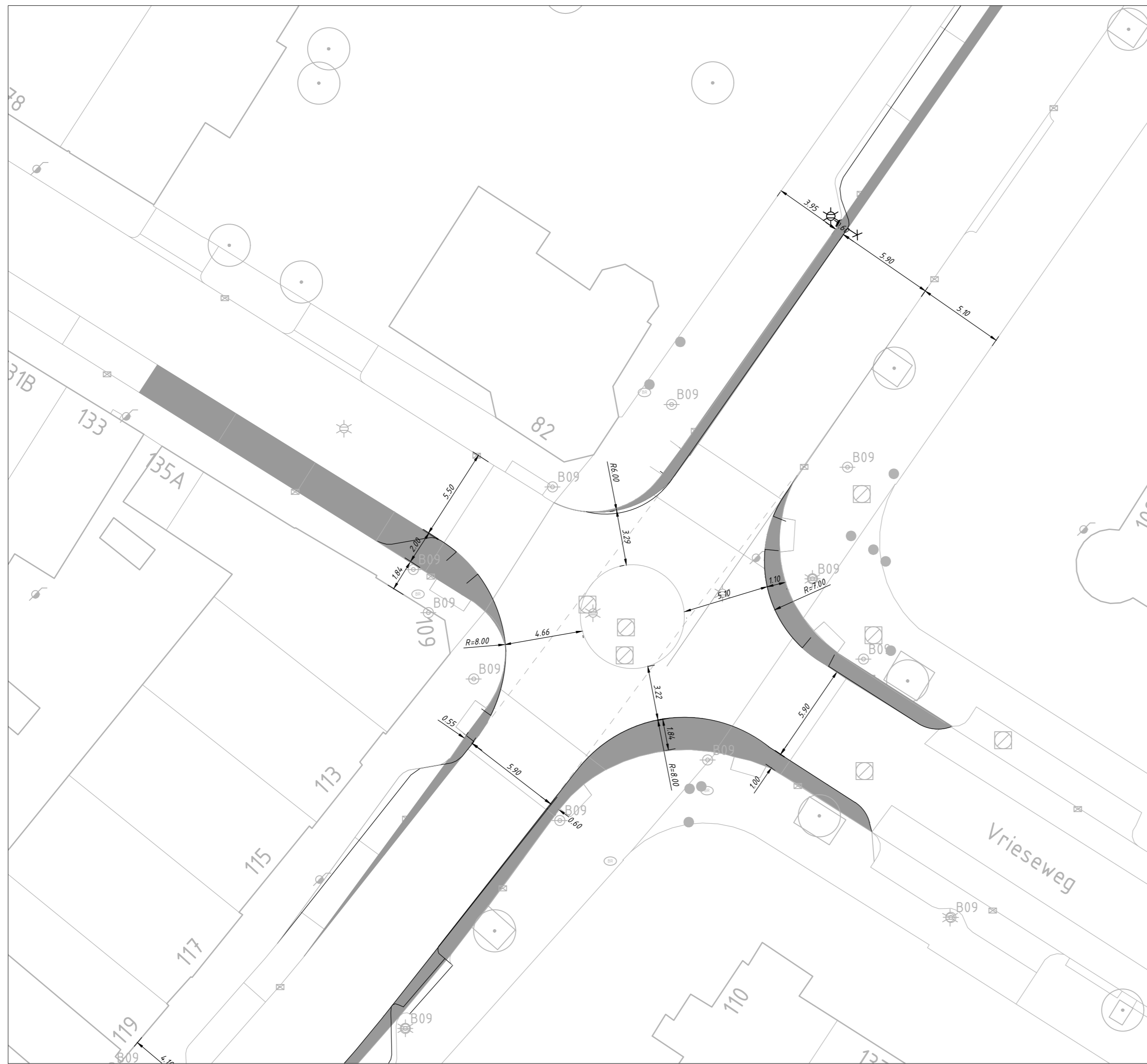
Kruising F. Bolsingel - S. van Hoogstratensingel schaal 1:200
