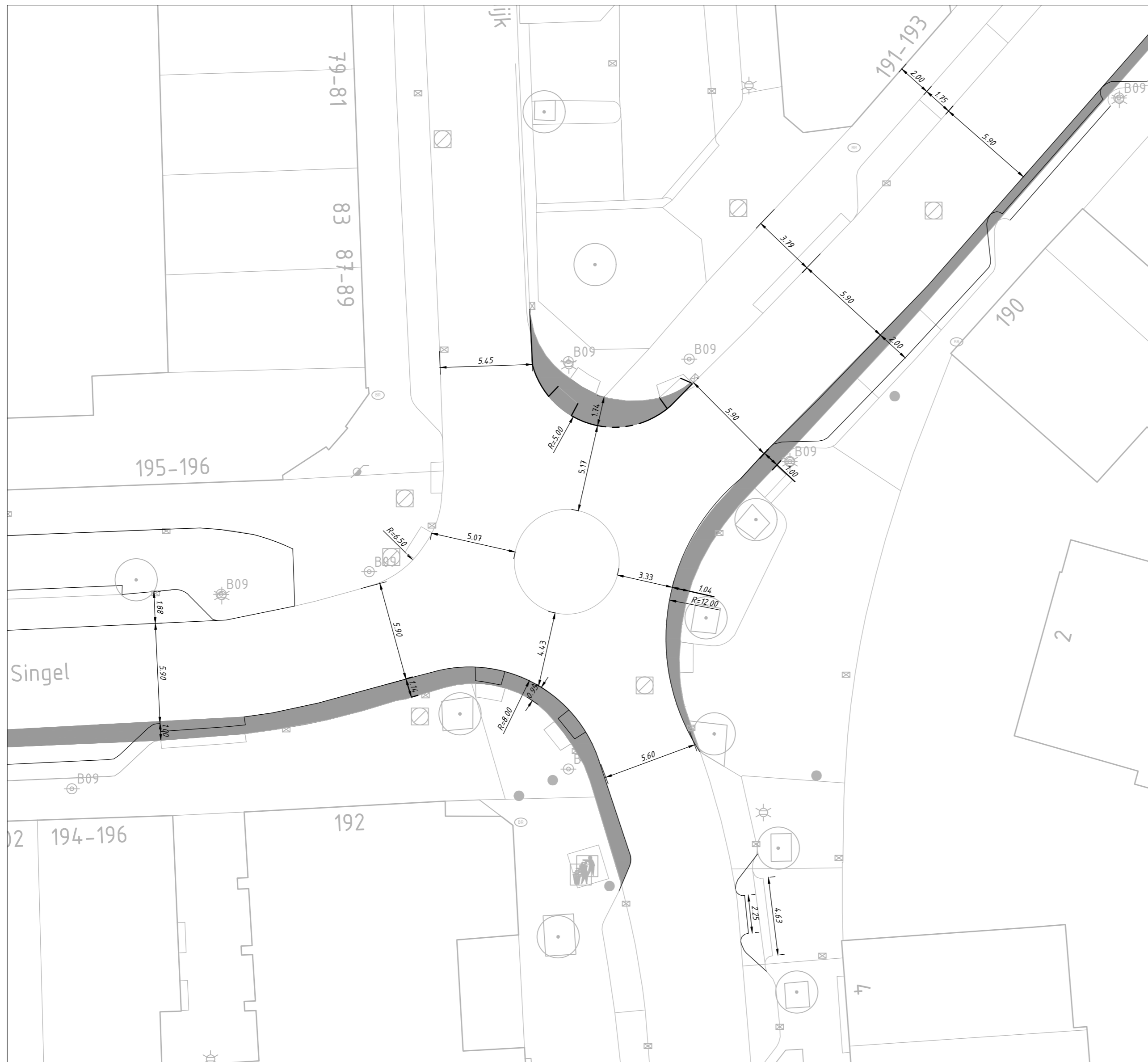
Kruising Nic. Maessingel - F. Bolsingel schaal 1:200
