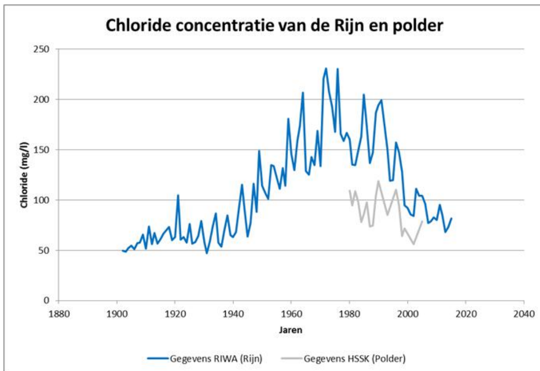
Figuur 9: Gemeten chloride concentratie in Rijnwater en polderwater. De gegevens zijn verzameld door het Hoogheemraadschap van Schieland en de Krimpenerwaard.
