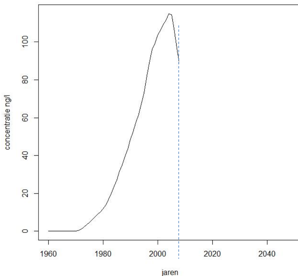
Figuur 19: Berekende concentratie PFOA in het ruwwater van Zwijndrecht voor de periode van 1960 tot 2009.
